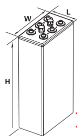
7 OPzS 700 - 12 OPzS 1500
