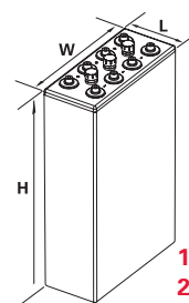
13 OPzS 1625 - 16 OPzS 2000
